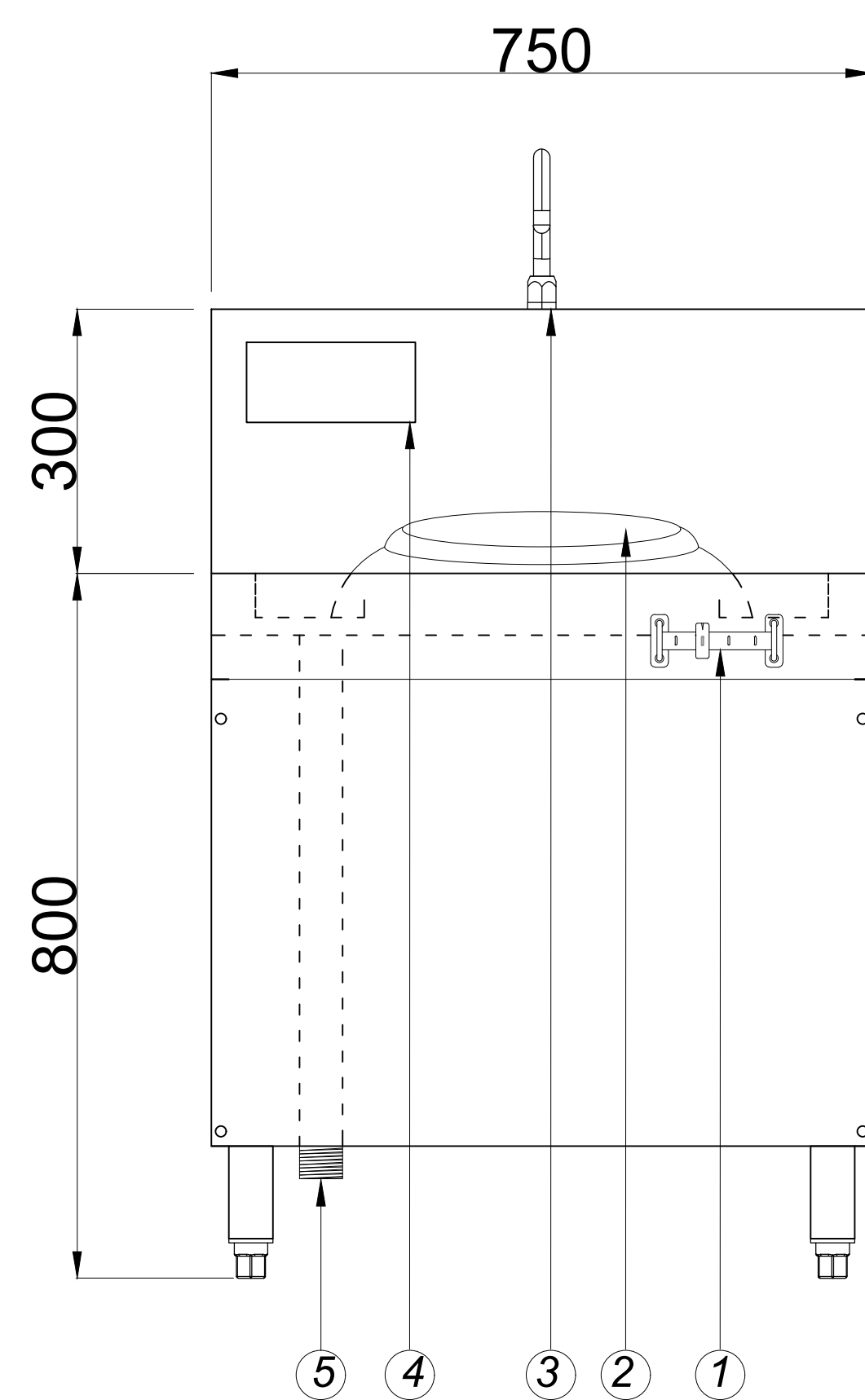
ELEVATION
